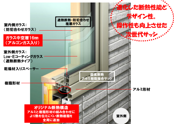
ワンランク上の高い意匠性と機能性を両立した 積水ハウスオリジナルの超高断熱サッシ
