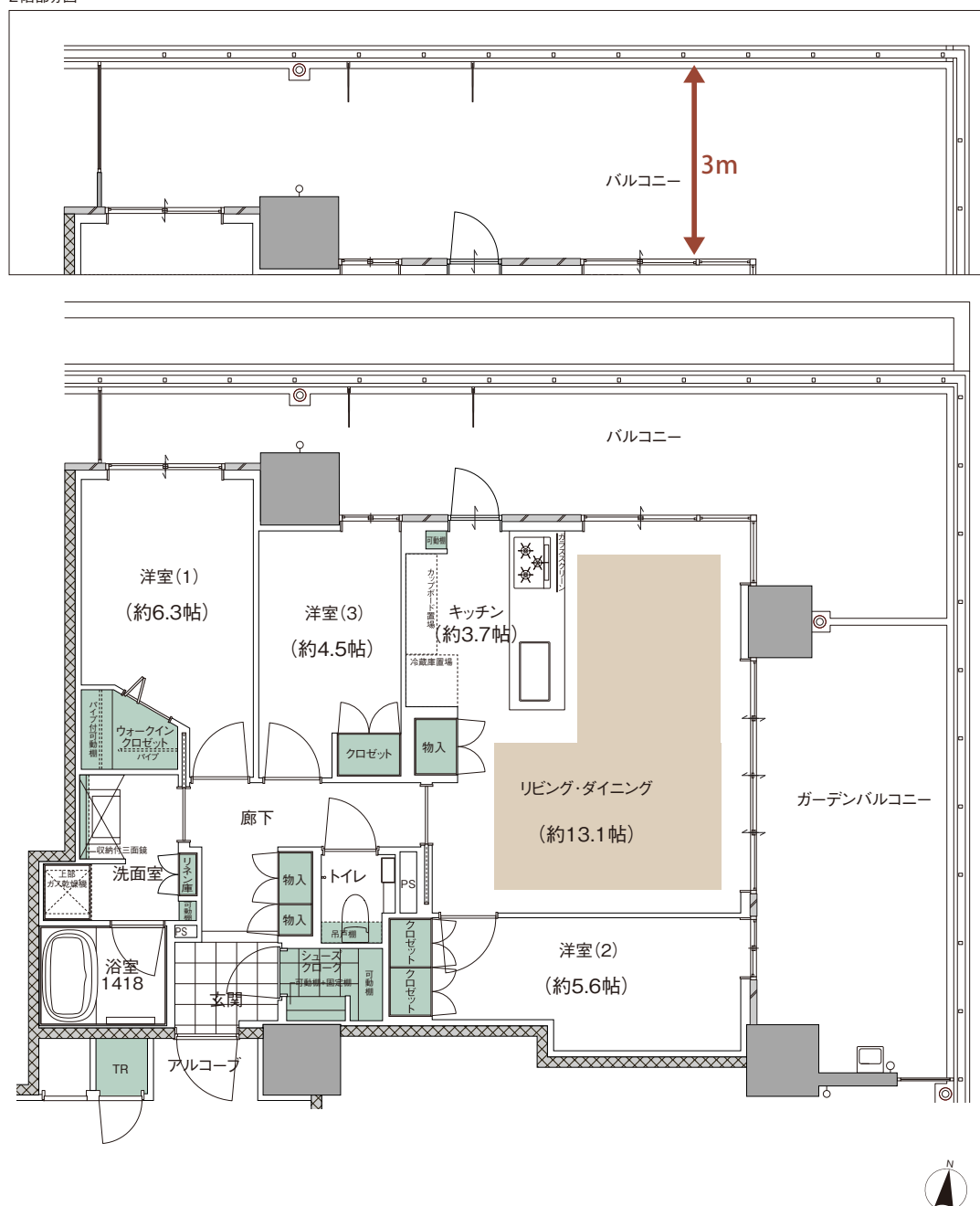
2階部分図
