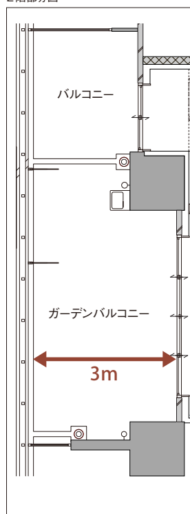
2階部分図
