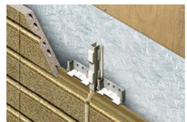
専用の金具により取り付け
